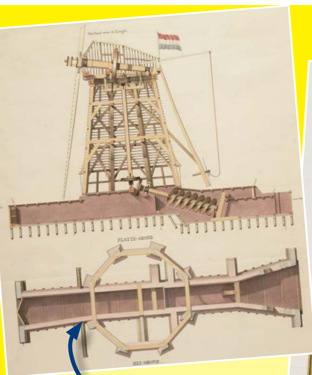
Waterrad Vijzel
