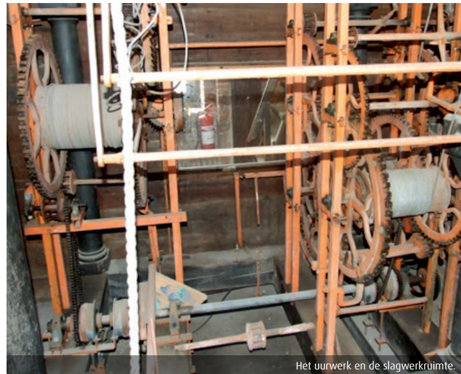
Het uurwerk en de slagwerkruimte.
