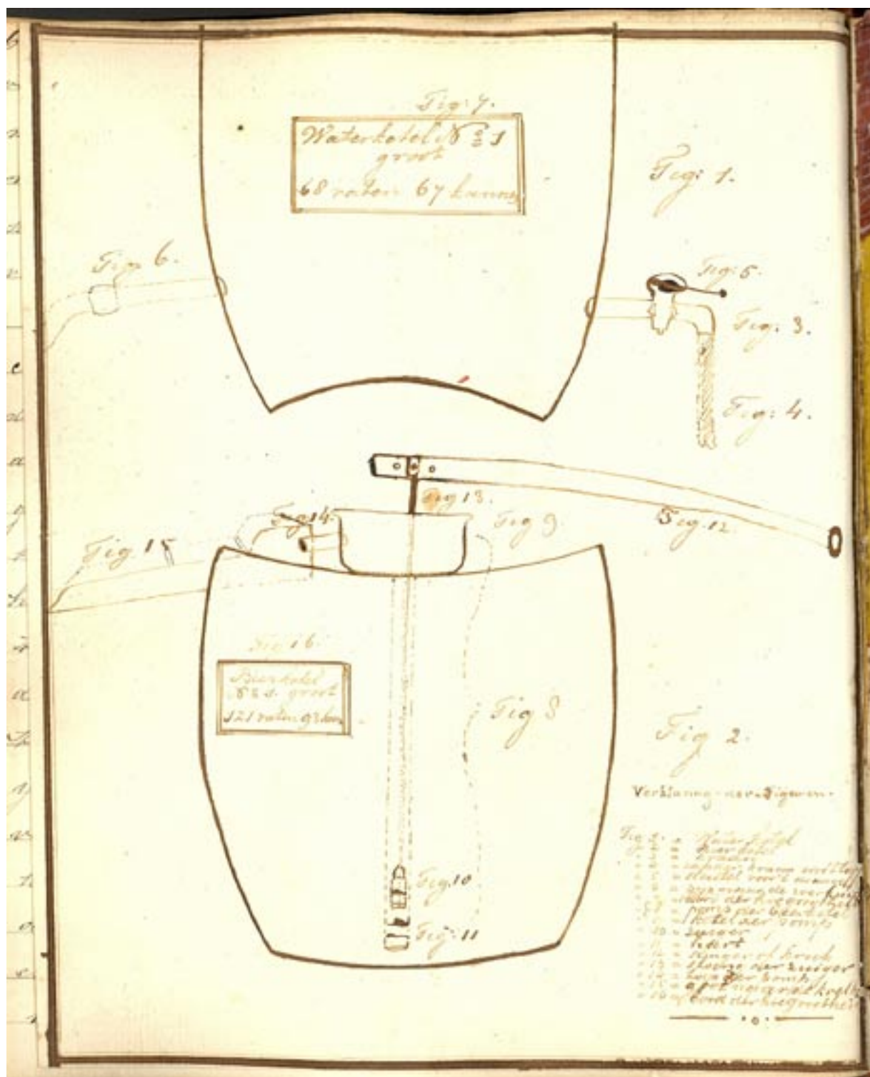
De warmwaterketel en de brouwersketel (J.J.G. Wahlen, 1862-1865) [Collectie Regionaal Archief Alkmaar]
