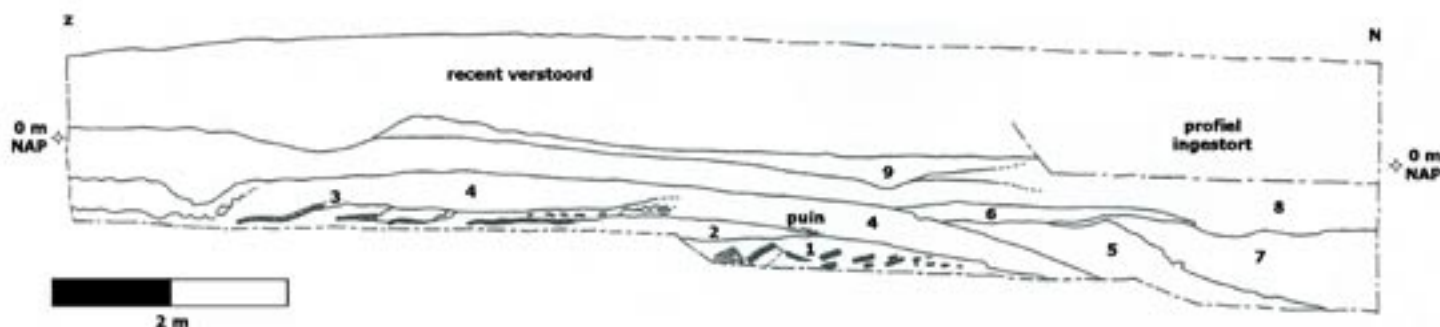
profiel 1 WP 4 zuiddeel
