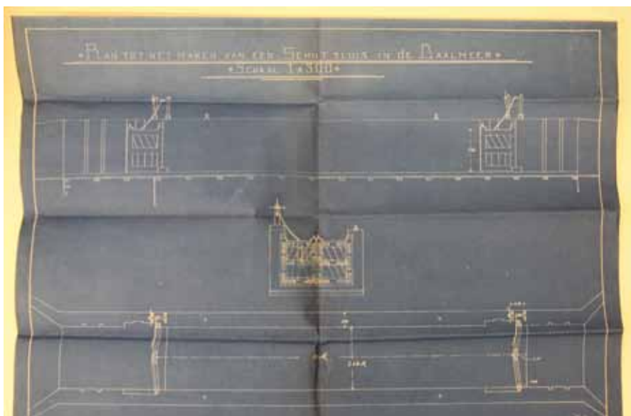
De plantekening van het sluisje dateert uit januari 1920. (Uit het archief van de Polder Daalmeer, in bewaring bij het Hoogheemraadschap Hollands Noorderkwartier)
