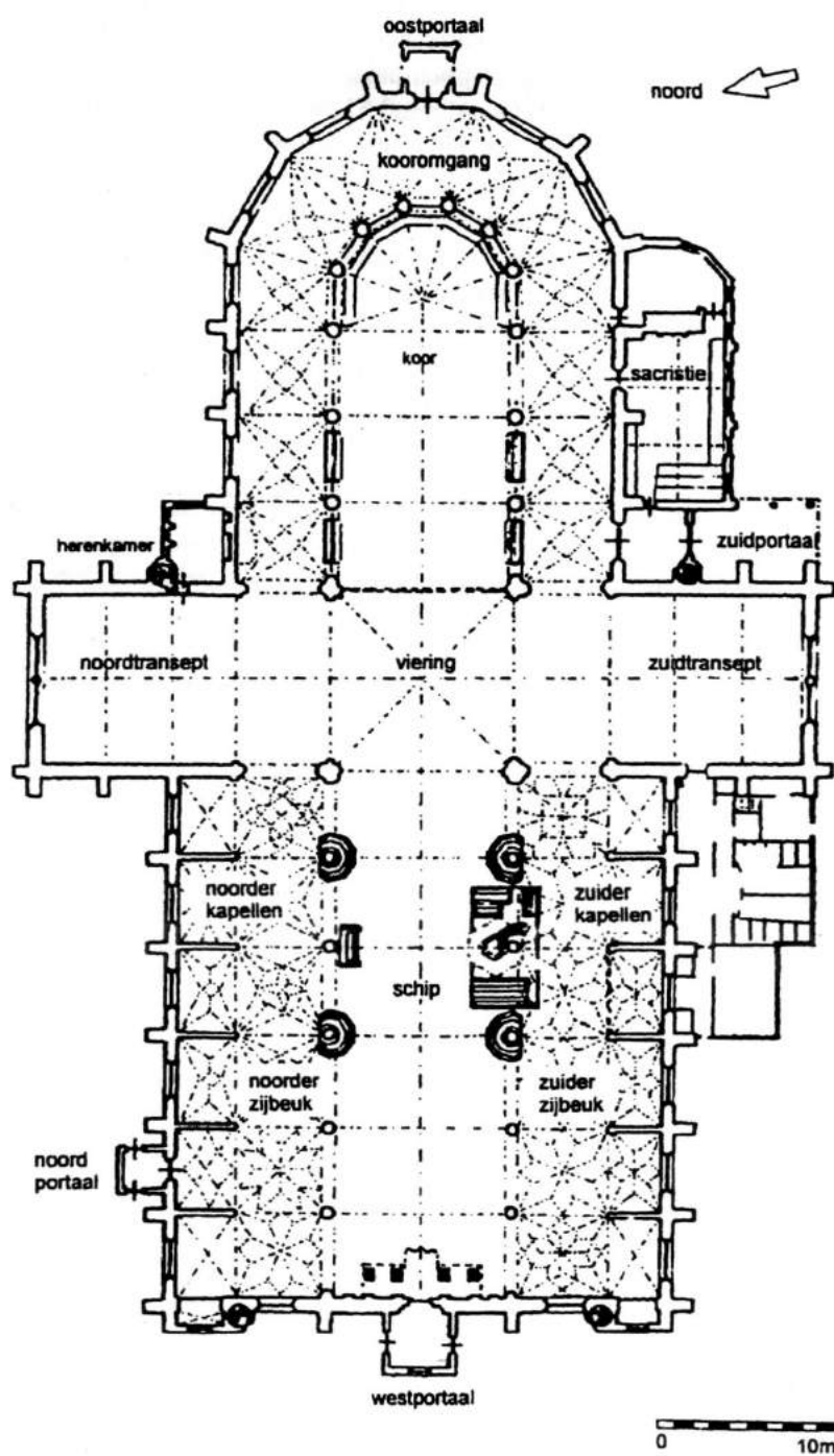
Plattegrond van de St. Laurenskerk
